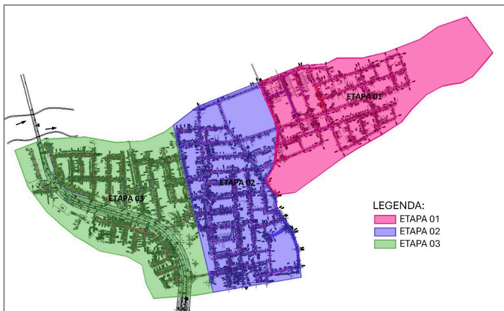
Figura 01: Projeto de Urbanização de Vila Canaã - Divisão das Etapas. Data:08/04/2025
