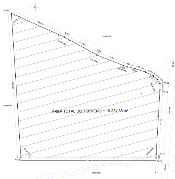
ETE Nazaré: Planta de Situação – sem escala.
