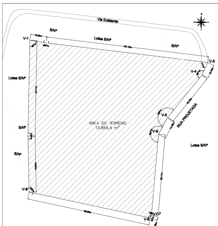
ETE Caetés: Planta de Situação – sem escala.
