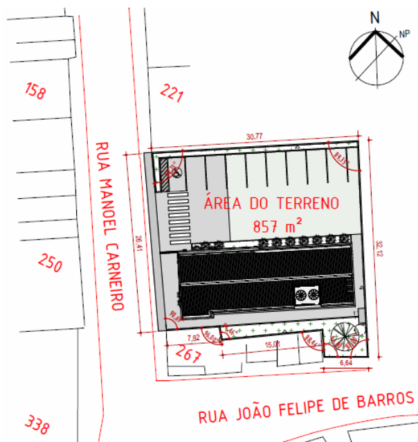
Araçoiaba: Planta de Situação – sem escala.
