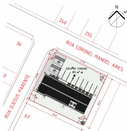
Exu: Planta de Situação – sem escala.
