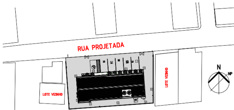
Casinhas: Planta de Situação – sem escala.
