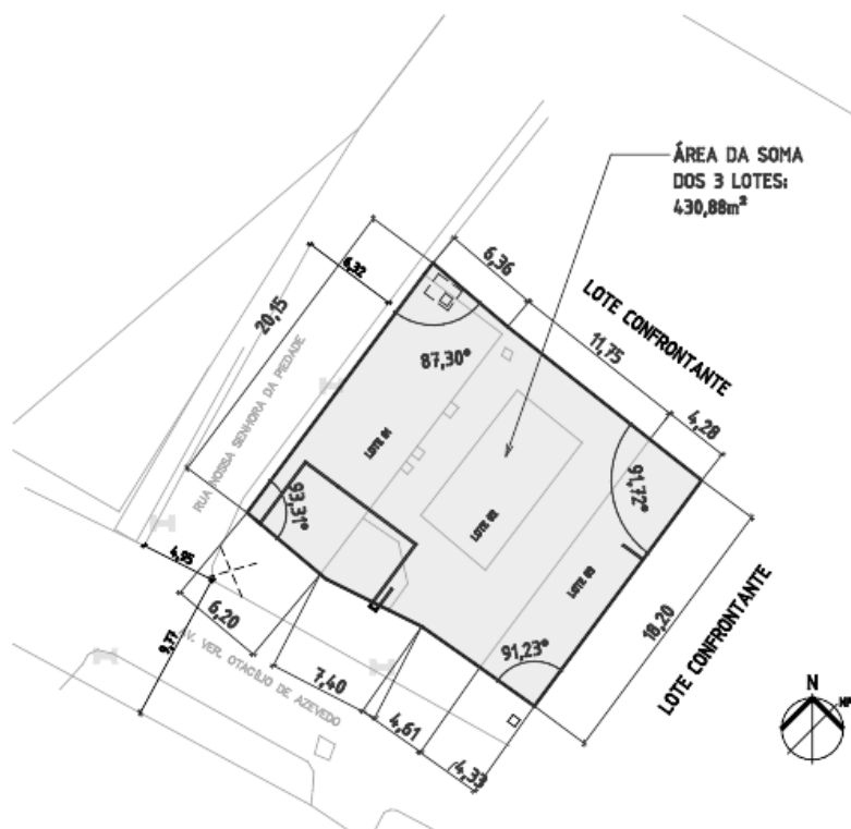
Delegacia de Polícia Civil - Nova Descoberta: Planta de Situação – sem escala.
